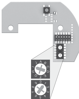
Drehschalter
