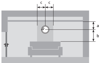
Wandmontage eines Rauchwarnmelders
